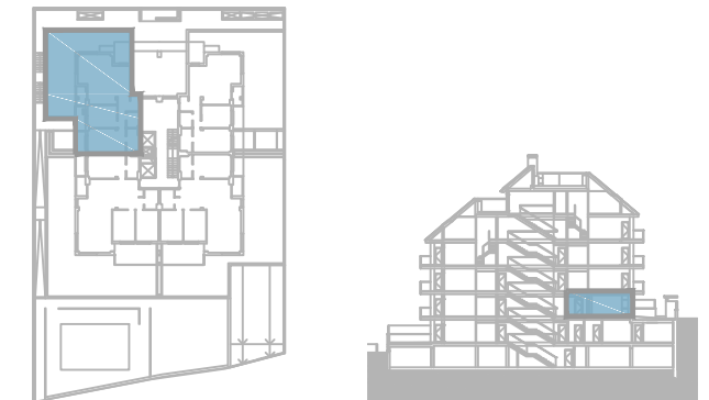
Viv. Tipo 03 _ Planta acceso Puerta A
